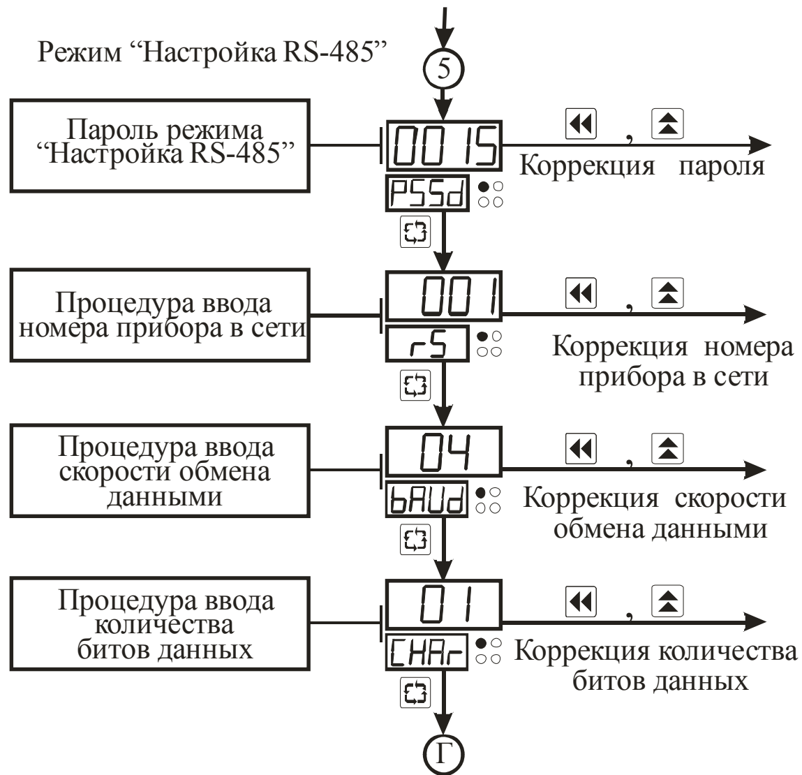
Рисунок 3.12 – Схема алгоритма работы в режиме “Настройка RS”
