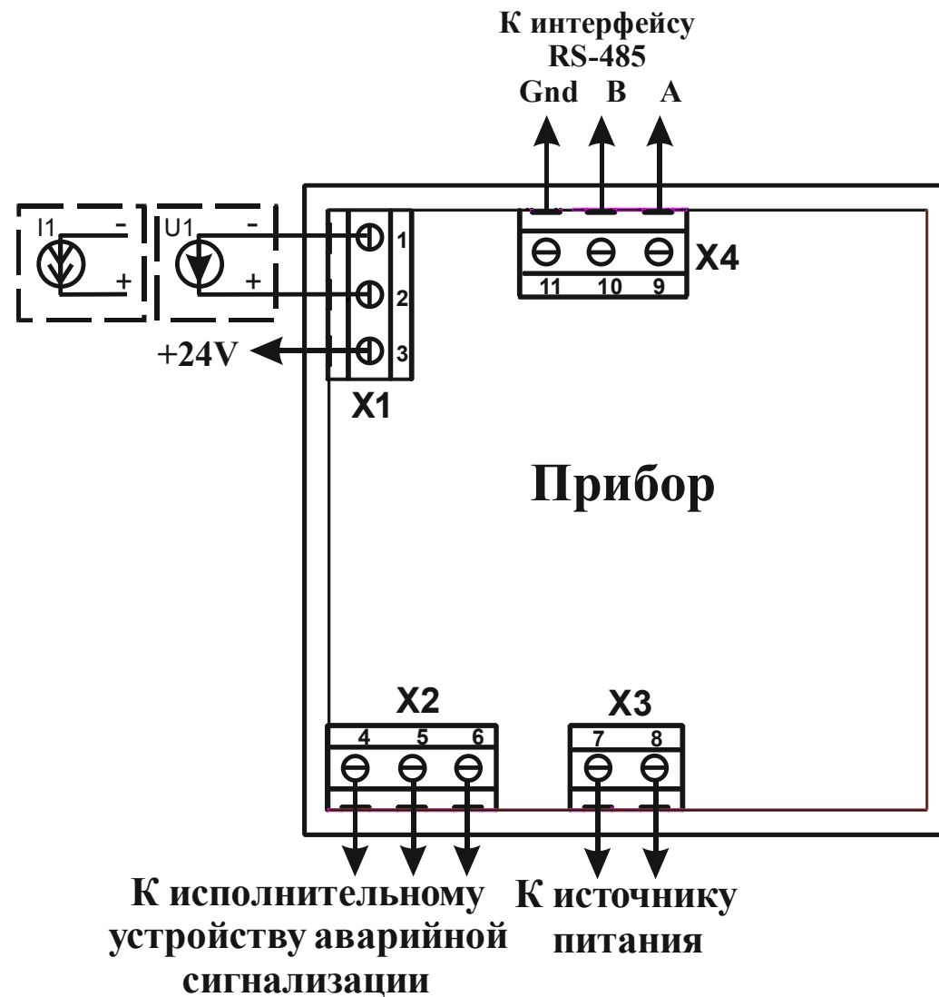
Рисунок 8.2 – Схема подключения датчика, источника питания, исполнительного устройства и интерфейса RS-485(модификация АН [АТ])
