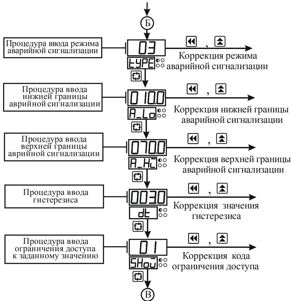
Рисунок 3.6 – Схема алгоритма работы в режиме “Коэффициенты” (продолжение)
