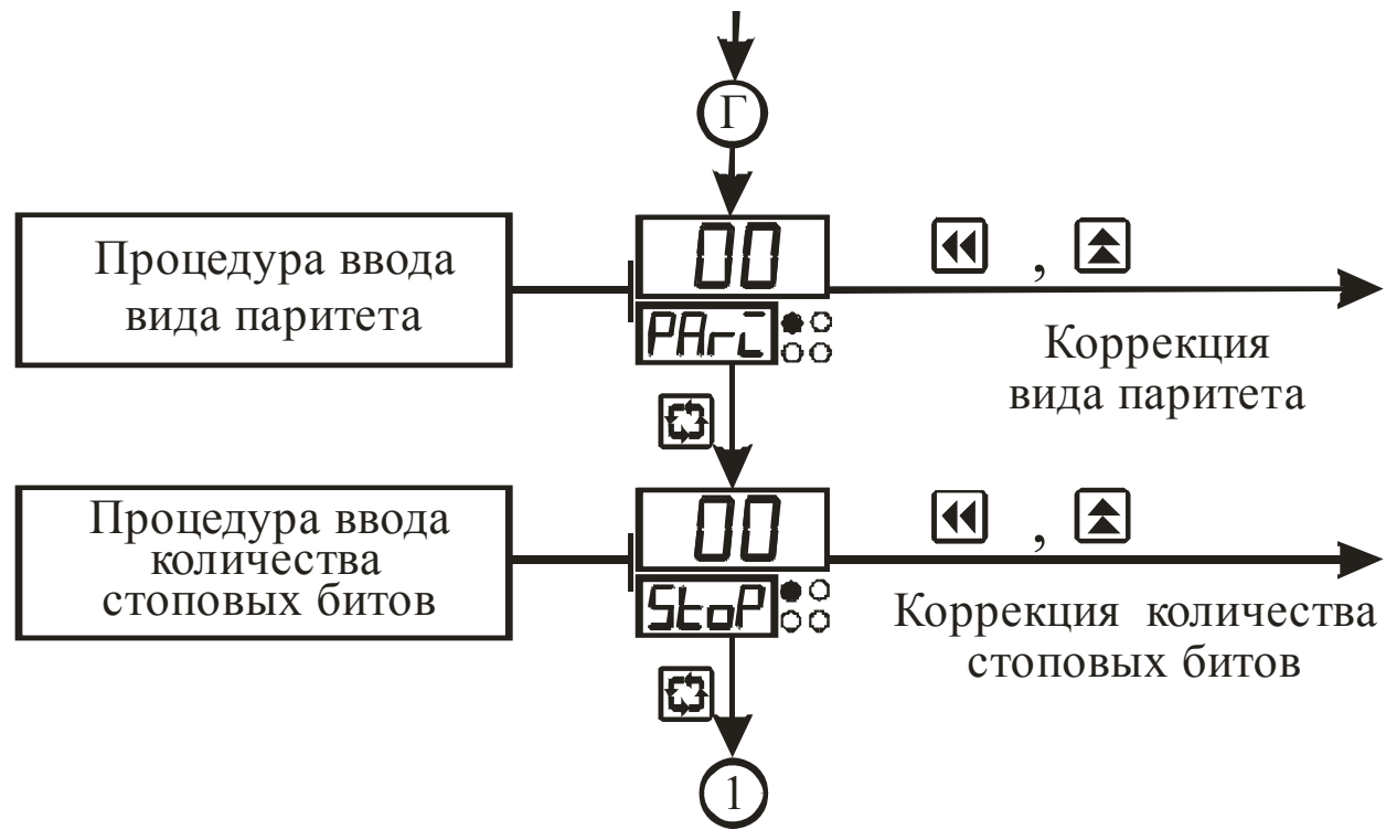
Рисунок 3.13 – Схема алгоритма работы в режиме “Настройка RS” (окончание)
