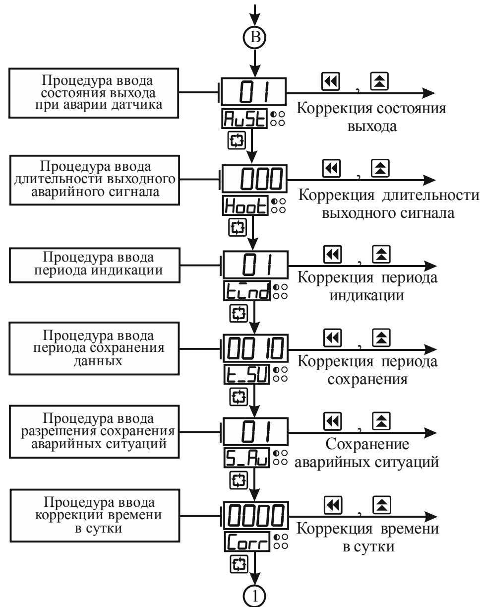
Рисунок 3.7 – Схема алгоритма работы в режиме “Коэффициенты” (окончание)
