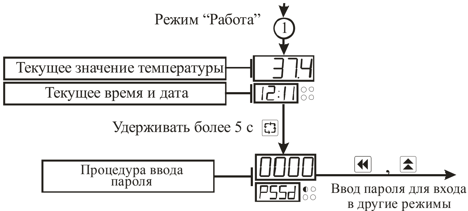
Рисунок 3.3 – Схема алгоритма работы в режиме “Работа”
