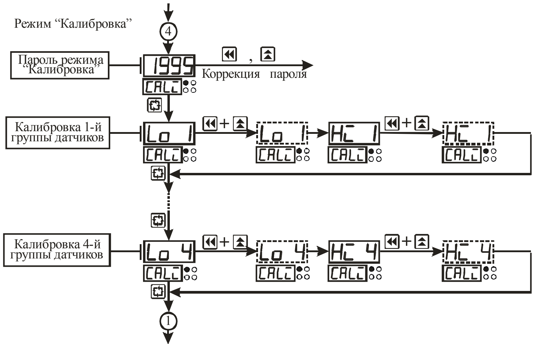
Рисунок 3.11 – Схема алгоритма работы в режиме “Калибровка”
