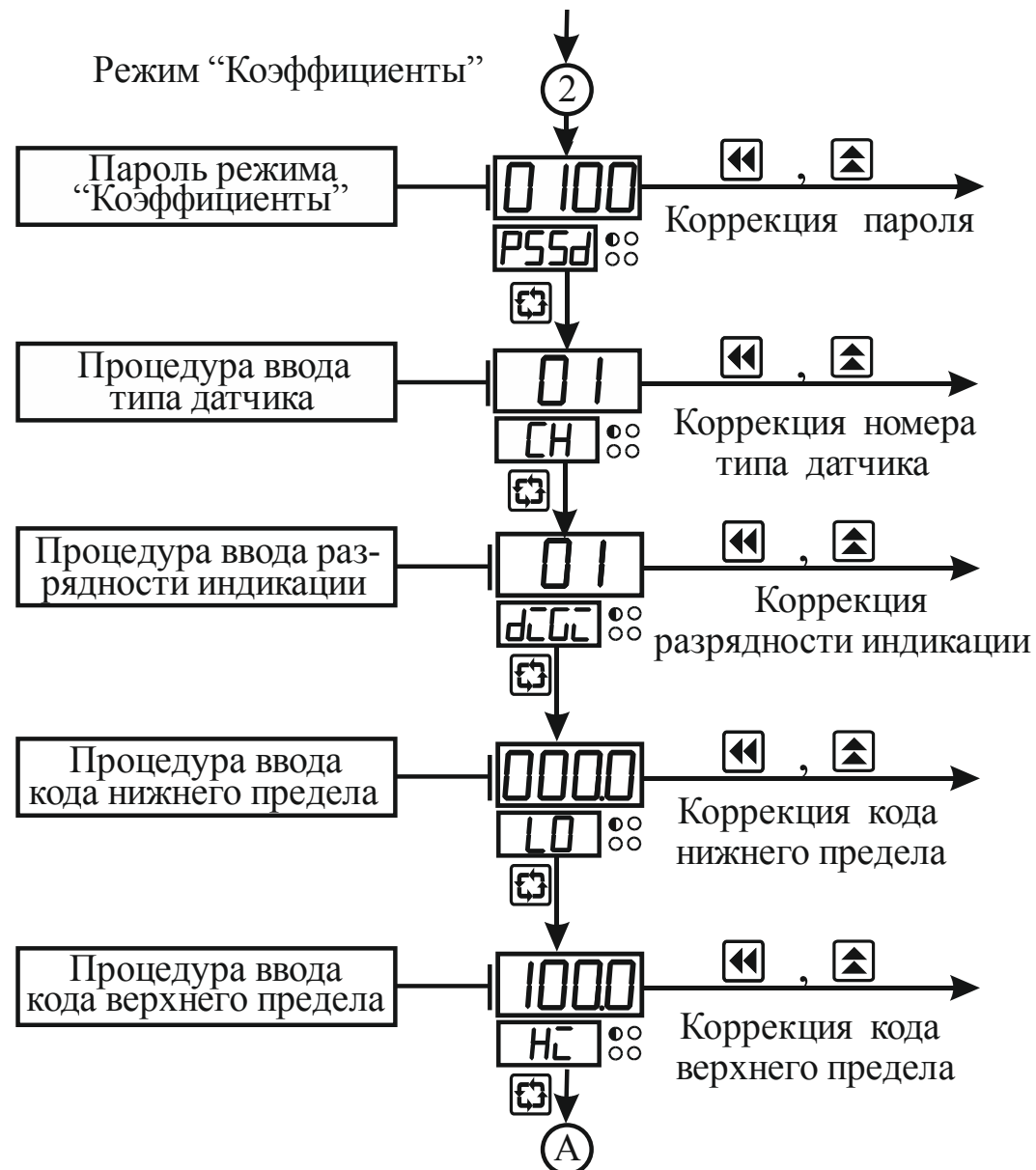
Рисунок 3.4 – Схема алгоритма работы в режиме “Коэффициенты”
